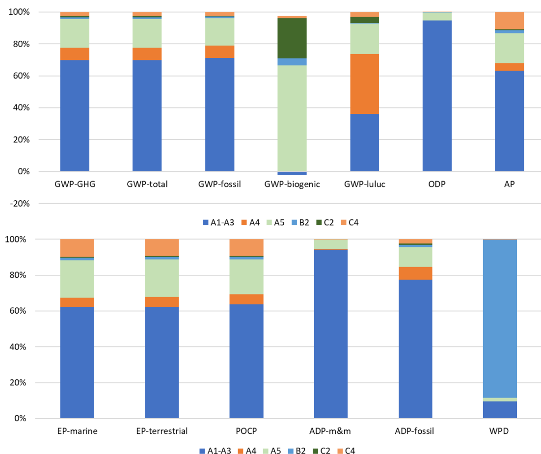
Figure 2. Contributions des différents modules relatifs aux catégories d'impact.
